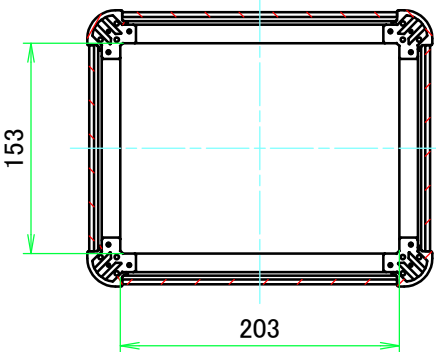
C-C ( 1 : 5.5 )
