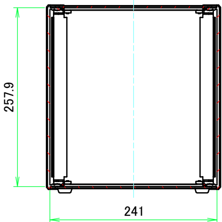
A-A ( 1 : 5.5 )
