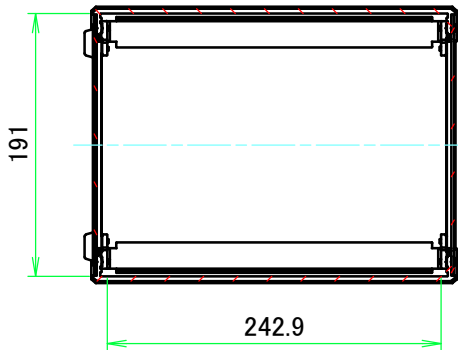
B-B ( 1 : 5.5 )
